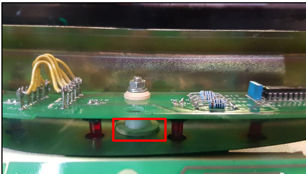
Imatge 2- Vista posterior del muntatge cap del cargol i volandera.
