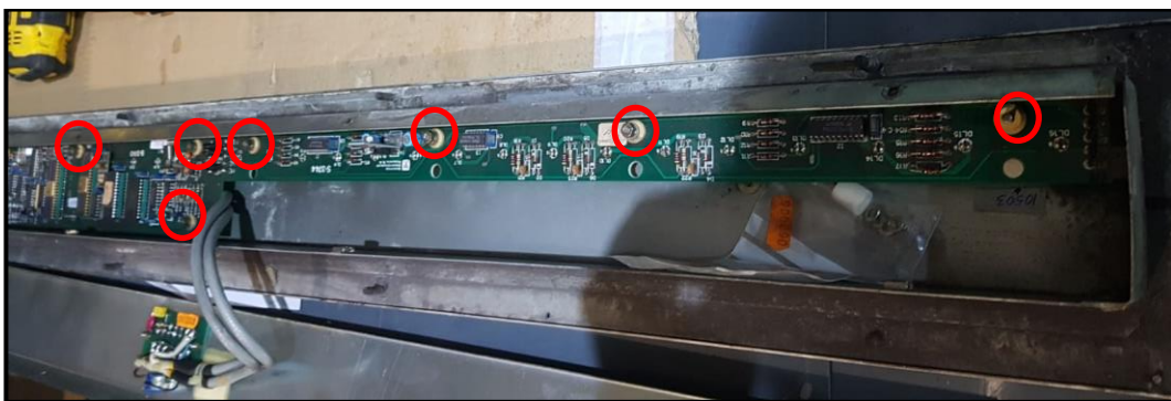
Imatge 1- La FAE 10.503 es troba entre el cap del cargol i la placa PCB. En aquesta imatge quedaria darrere de la PCB on estan les marques vermelles.
