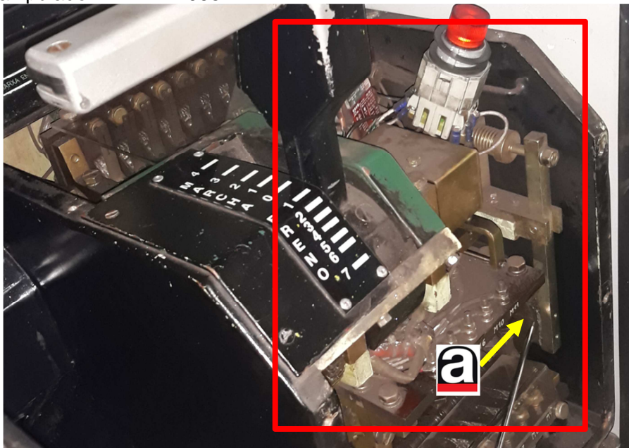
Imagen 1. Localización del ferodo del manipulador en el pupitre de mando.
